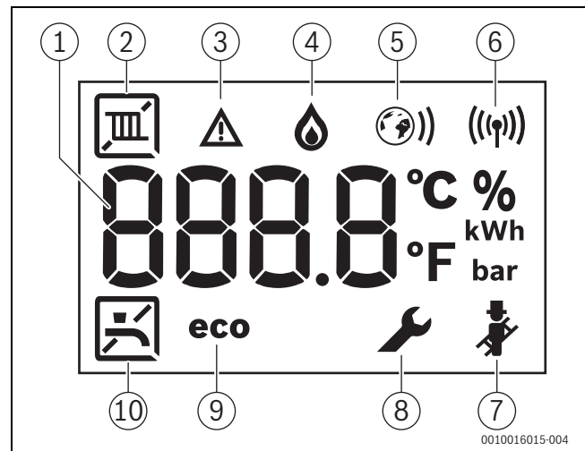
Fig. 7 Screen display
